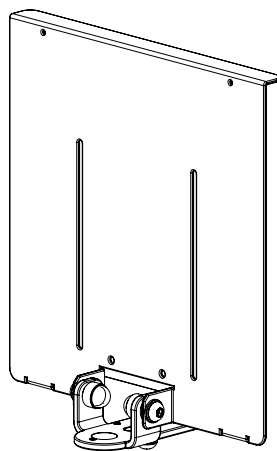
Laptop bracket Art.-Nr. 961330 1pcs
